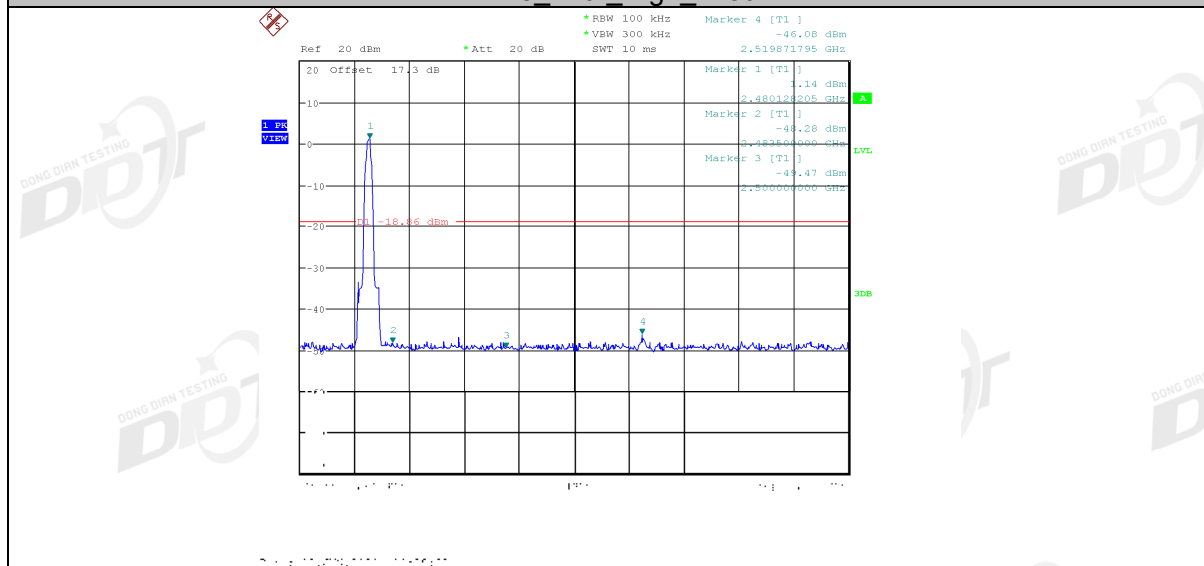
2DH5_Ant1_Low_Hop_2402
